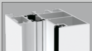
Pravouhlé vyhotovenie (profil A2)
